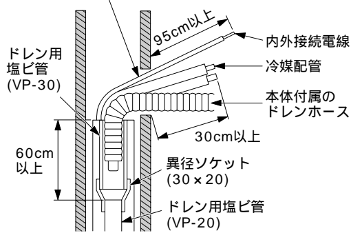
壁の内部を横から見た図
