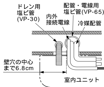
壁の内部を上から見た図
