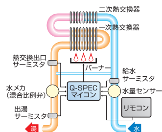
Q-SPEC制御図
