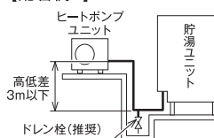
【配管例1】
