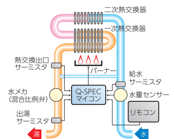
Q-SPEC制御図
