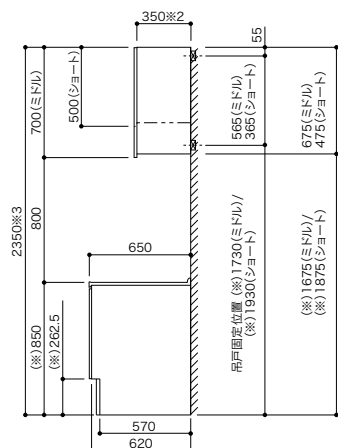
●側面図(H500・H700)
