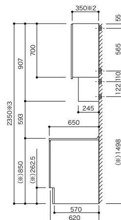
●オープンウォール (ミドルウォールと組み合わせた場合)
