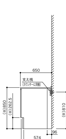
●コーナーキャビネット
