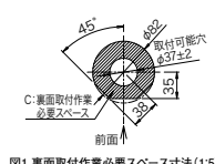
図1 裏面取付作業必要スペース寸法 (1/5)
