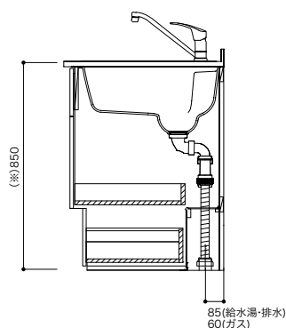
●側面図
