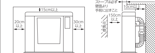
埋込設置図 FFR-703SX
