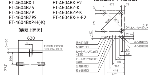
【機器上方よりの透視図】
