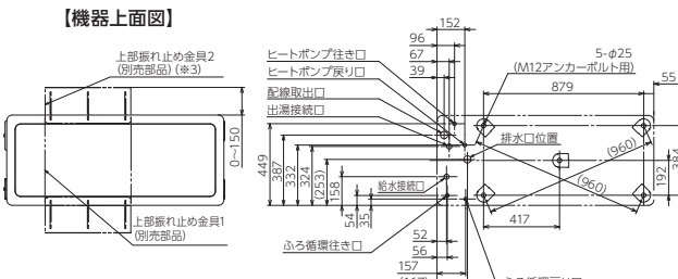
【機器上方よりの透視図】
