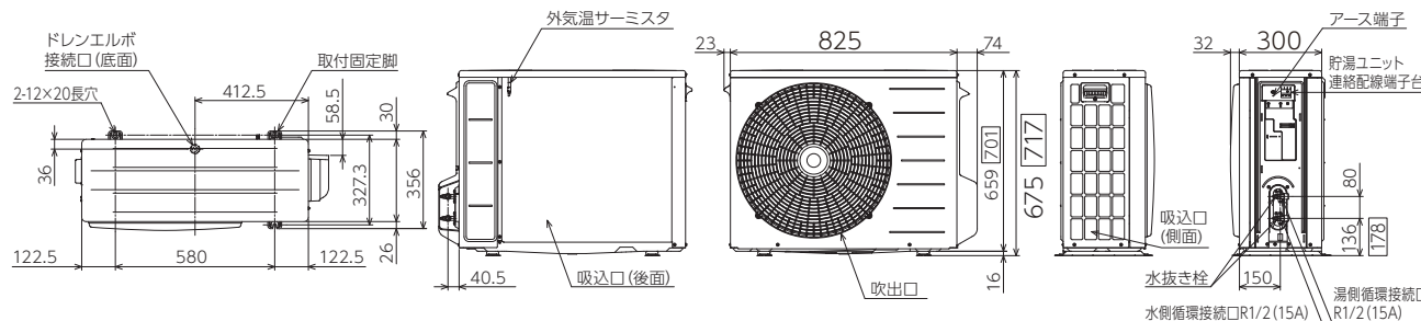
【配管カバー取外し時】
