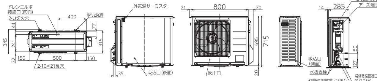
【配管カバー取外し時】
