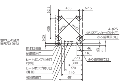
【機器上方よりの透視図】
