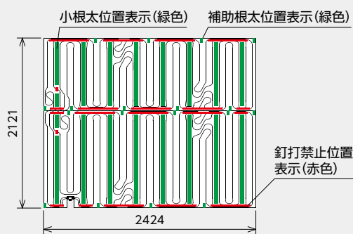
仕様図
