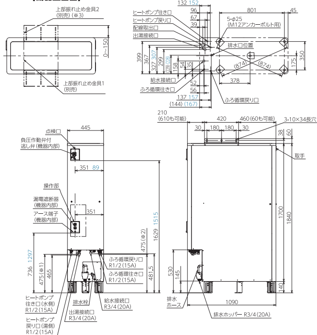
【機器上面図】
