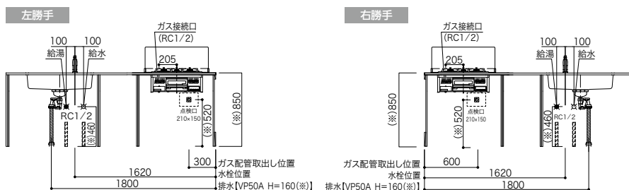
●側面図
