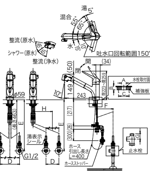
図1 裏面取付作業必要スペース寸法
