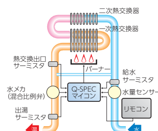
Q-SPEC制御図
