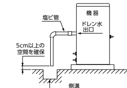
側溝へ排水する場合
