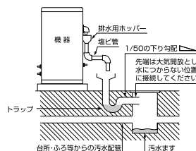
側溝へ排水する場合
