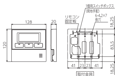
リモコン寸法図 (単位:mm)
