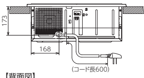
【背面図】
