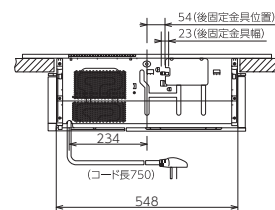
【背面図】
