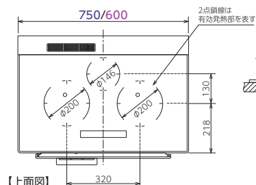
【上面図】
