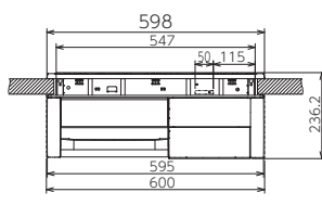
【正面図】
