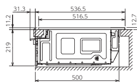
【側面図】
