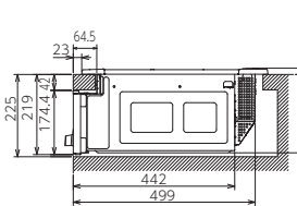
【側面図】
