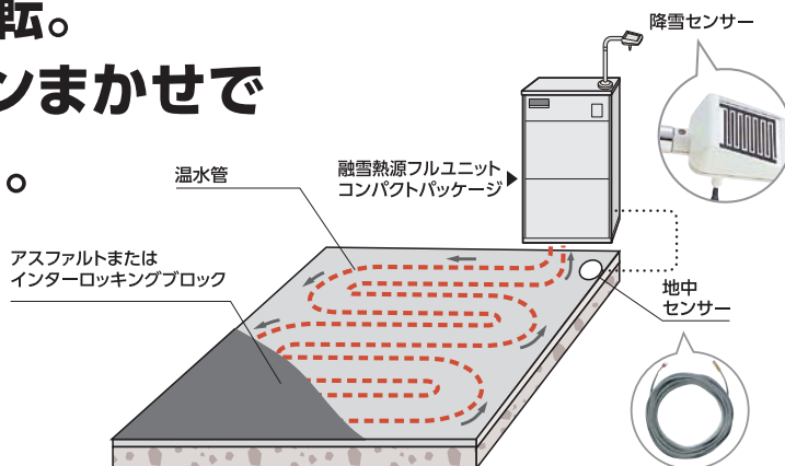
<温水ロードヒーティング システム図>
