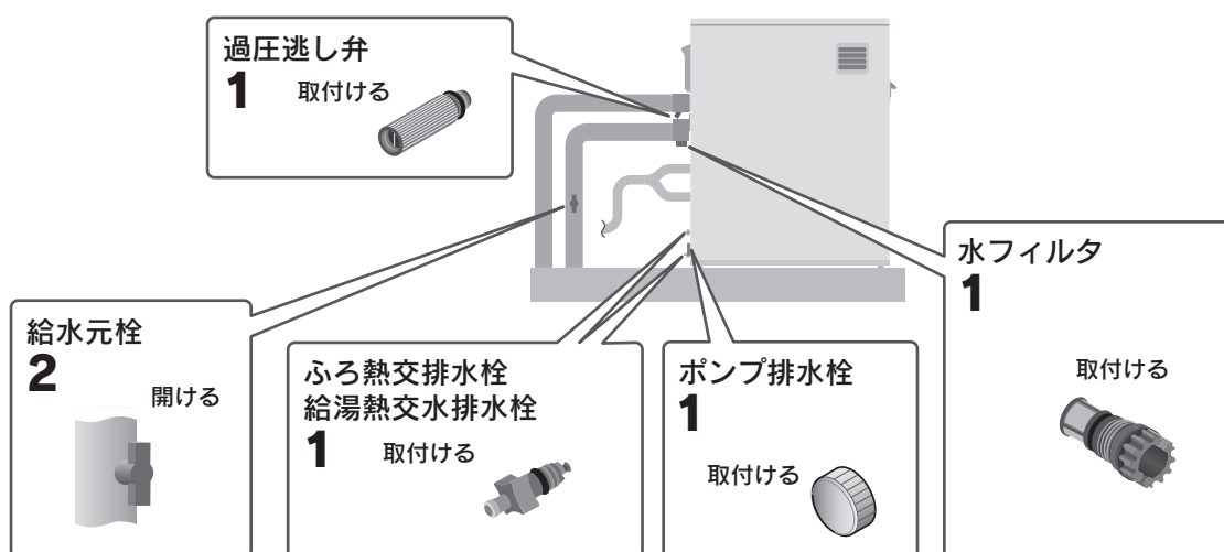
床置型 (前面排気タイプ)
