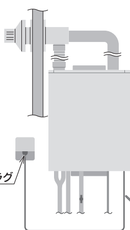
壁掛型 (強制給排気タイプ)
