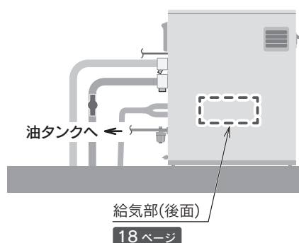
床置型 (前面排気タイプ)
