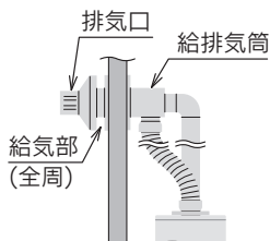
強制給排気タイプ
