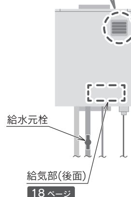
壁掛型 (前面排気タイプ)
