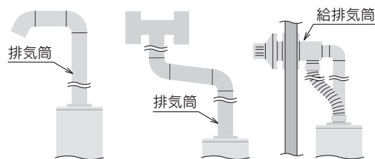
強制排気タイプ
