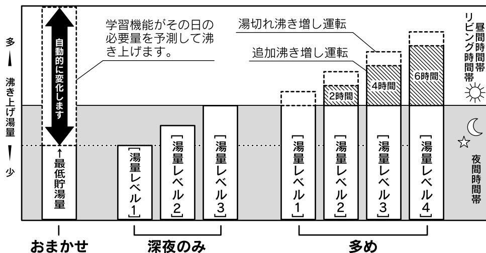
沸き上げ設定と沸き上げ湯量の関係
