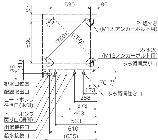
【機器上方よりの透視図】
