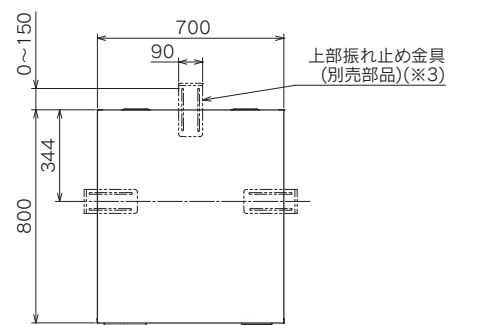
【機器上面図】
