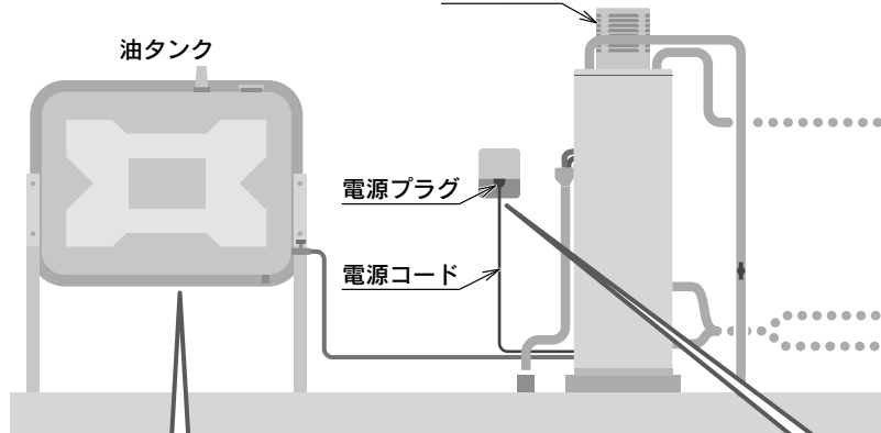
無煙突タイプ 拡散排気筒
