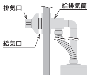
強制給排気タイプ
