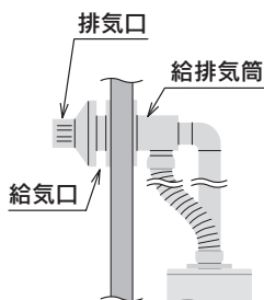
強制給排気タイプ
