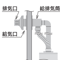
強制給排気タイプ
